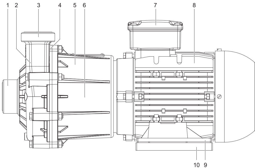
Abb. 3 Aufbau NHM
