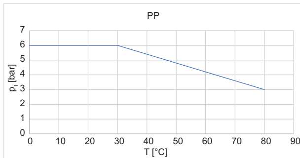
Abb. 9 Gesamtdruck, Werkstoff Pumpenkopf PP
